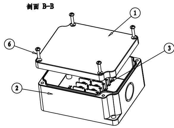
装配6位端子 比例 3:5
